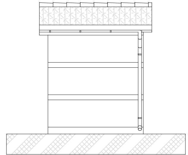
SEZIONE LONGITUDINALE
