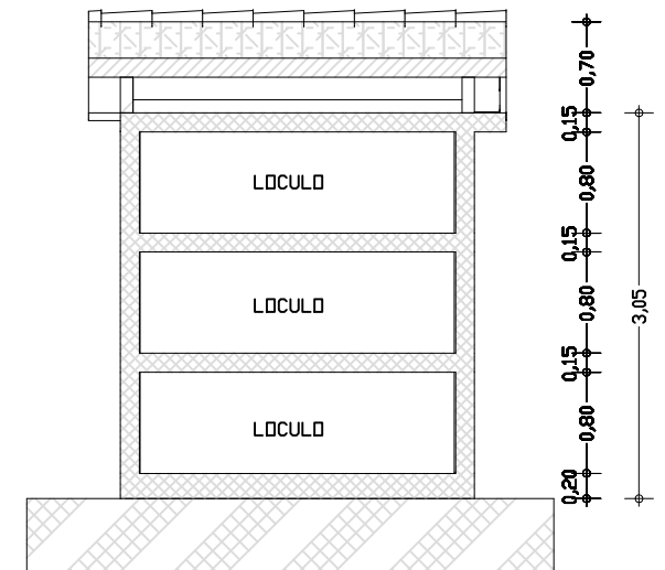
SEZIONE LONGITUDINALE
